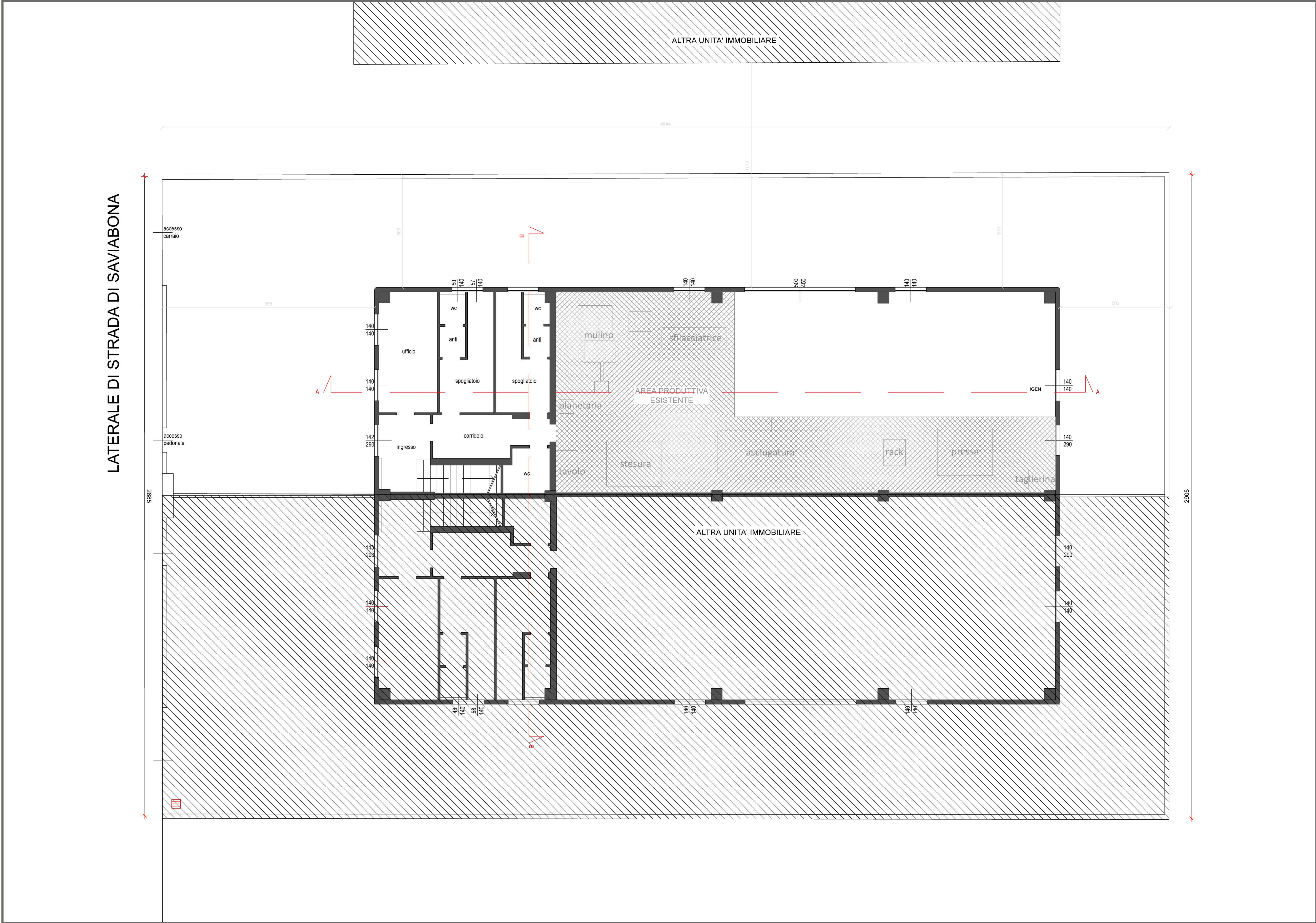
PIANTE - Stato di fatto - piano terra - scala 1 a 100
