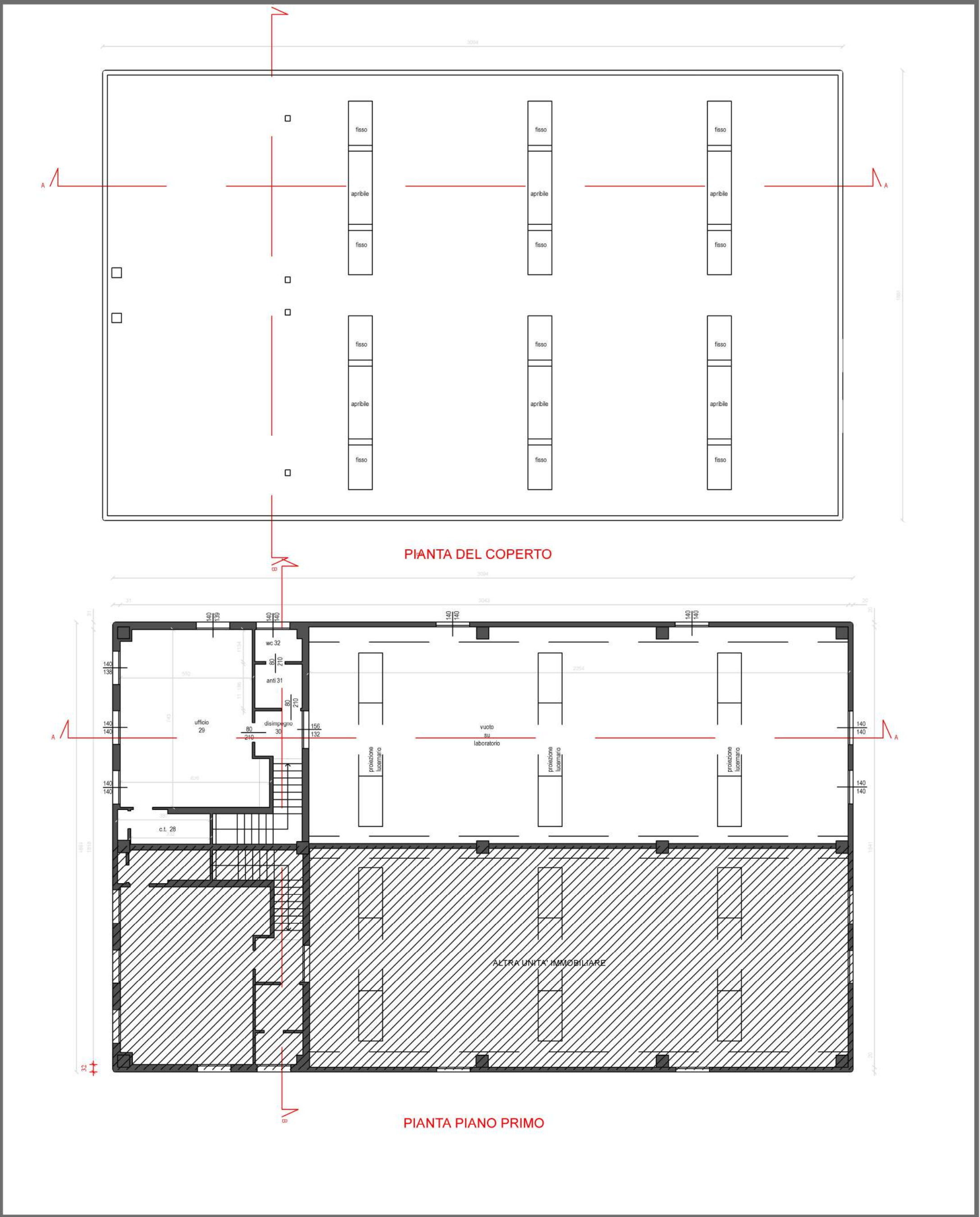
PIANTE - Stato di fatto - piano primo e copertura scala 1 a 200
